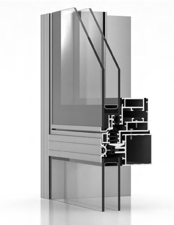
Вариант со штапиком
